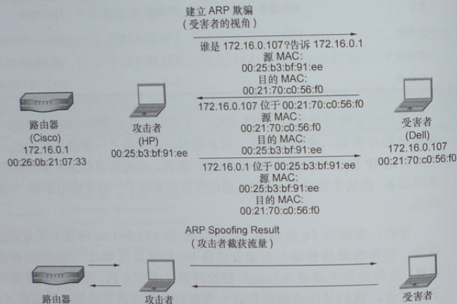
图 10-17 ARP 欺骗导致 MITM 攻击
