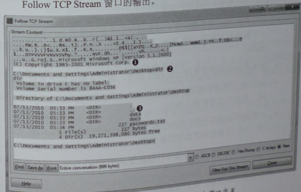
图 10-14 攻击者通过这个连接与命令窗口交互
