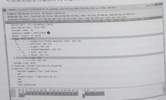
图 6-21 初始 SYN 数据包
