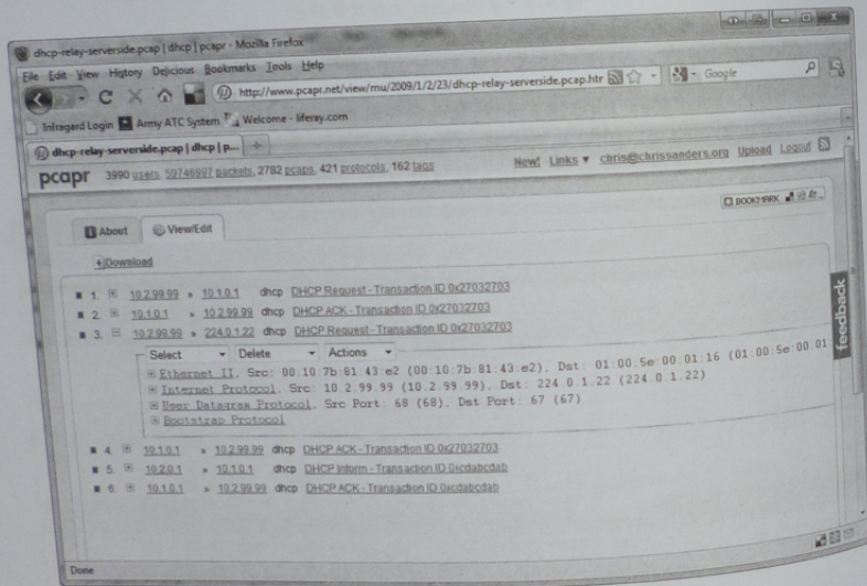
图 A-3 在 pcapr 上查看 DHCP 流量捕获
