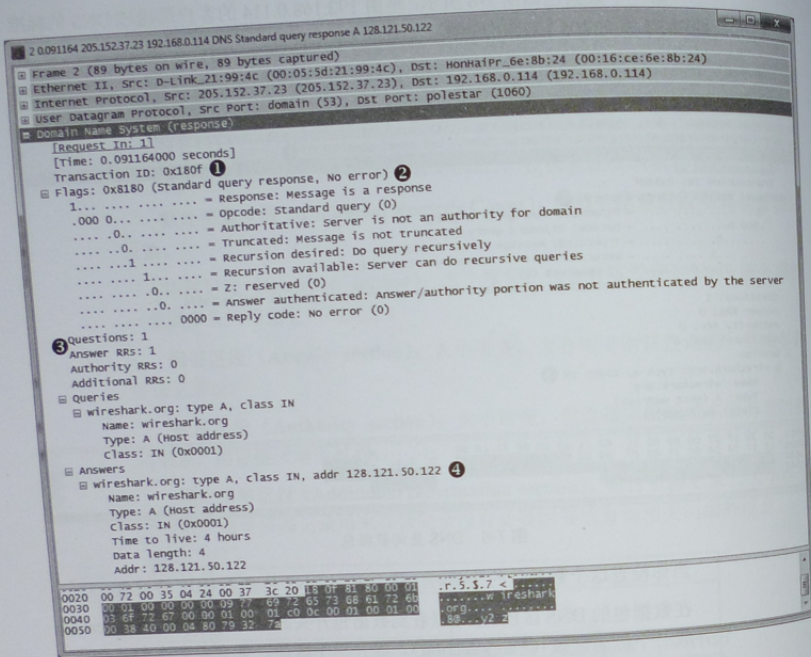
图 7-9 DNS 响应数据包
