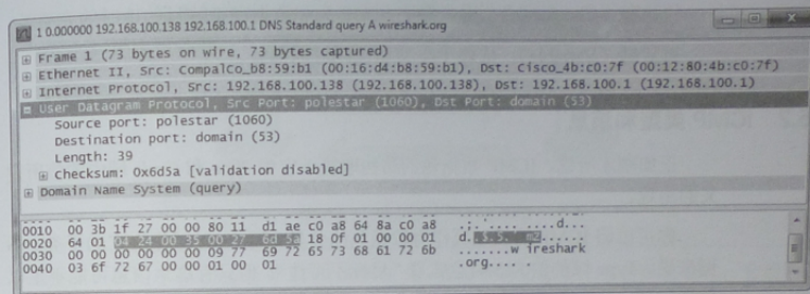
图 6-28 UDP 数据包的内容非常简单
