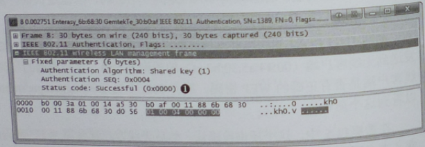
图 11-13 WAP 通知客户端认证成功
