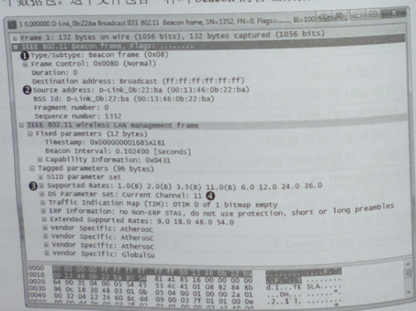
图 11-9 这是一个 802.11 beacon 数据包
