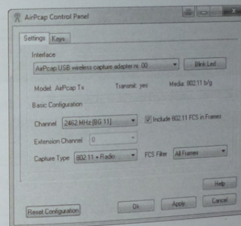
图 11-6 AirPcap 配置程序
