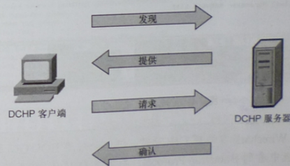
图 7-2 DHCP 的 DORA 过程
