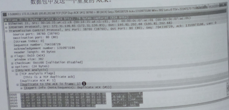
图 9-10 第一个重复 ACK 数据包
