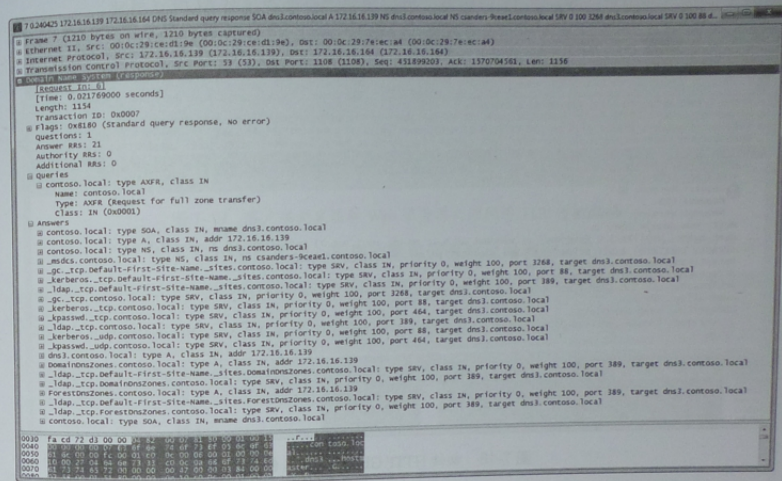
图 7-17 正在进行的 DNS 完整区域传送
