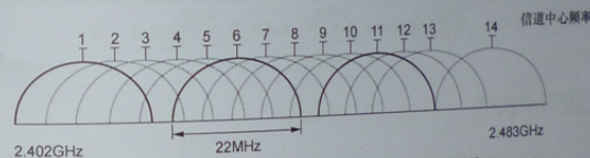
图 11-2 由于频谱空间有限，信道之间有重叠
