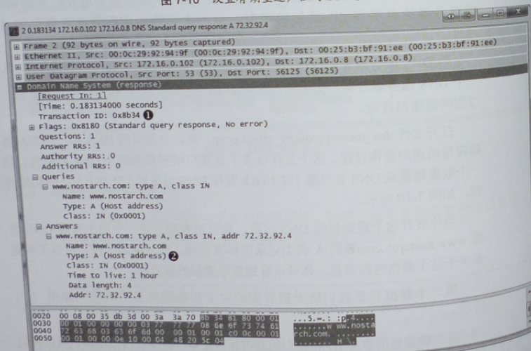
图 7-11 DNS 查询响应
