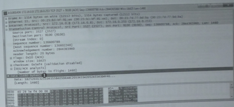
图 8-29 通过 TCP 传输到打印机的数据
