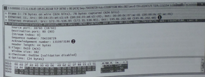
图 9-8 ACK 显示了下一个期待的序号
