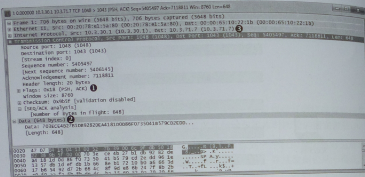
图 9-2 包含数据的简单 TCP 数据包
