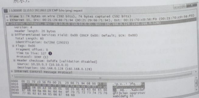
图 6-12 IP 头告诉我们 TTL 已经被减 1 了
