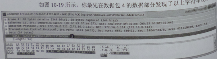
图 10-19 在数据包 4 中发现了 Snort 警报中的字符串内容
