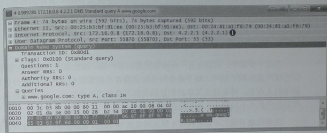
图 8-19 发送到 4.2.2.1 的第二个 DNS 查询
