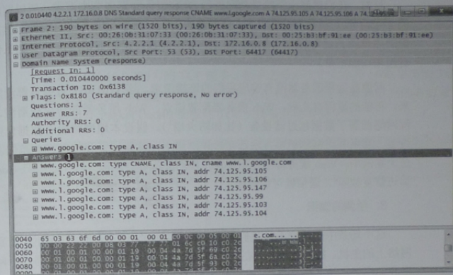
图 8-26 包含多个 A 记录的 DNS 响应
