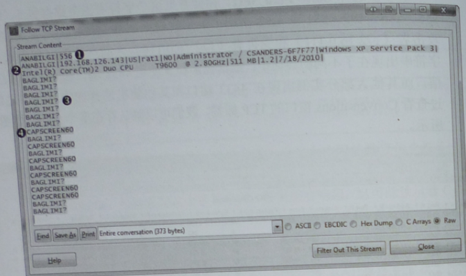
图 10-21 第一个会话产生了有趣的结果
