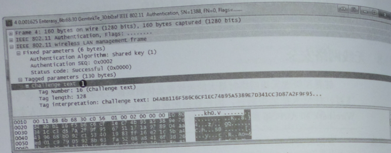
图 11-11 WAP 给无线客户端发送质询文本
