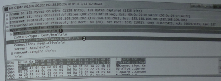
图 10-9 客户端浏览器被这个数据包重定向
