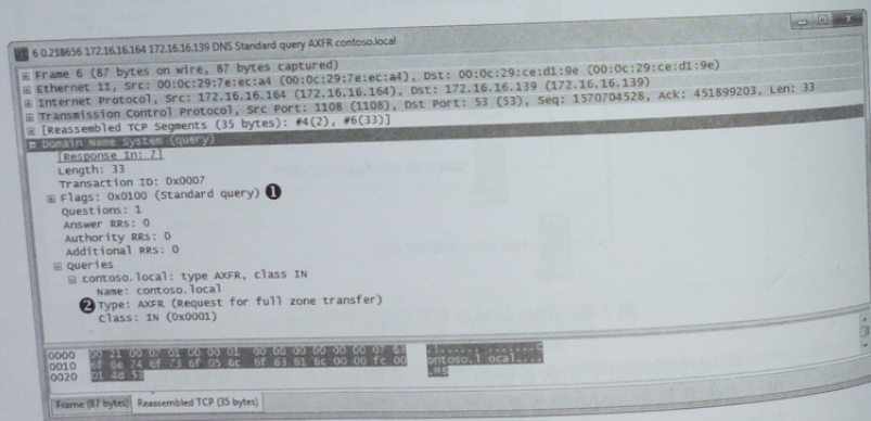
图 7-16 DNS 完整区域传送请求
