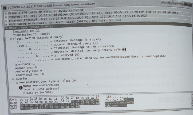
图 7-10 设置有期望递归位的 DNS 查询
