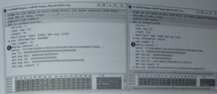
图 11-18 Replay Counter 域帮助我们匹配质询和响应
