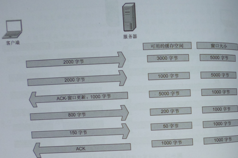
图 9-14 服务器变繁忙时，可以调整窗口大小
