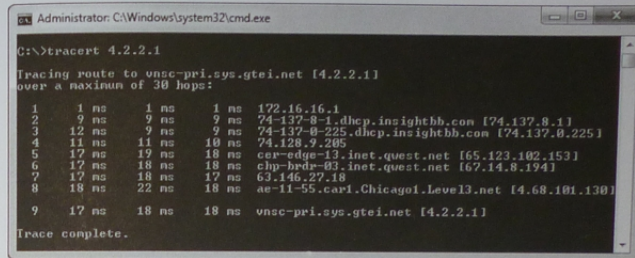
图 6-36 路由跟踪功能的样例输出
