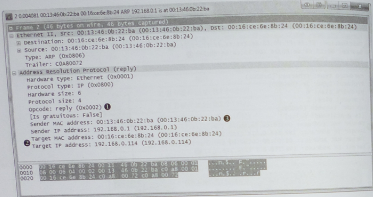
图 6-4 一个 ARP 回复数据包
