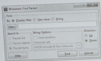
图 4-3 在 Wireshark 中根据条件查找数据包
