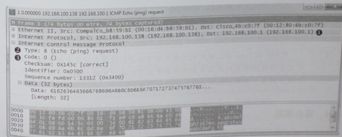
图 6-32 ICMP echo 请求数据包
