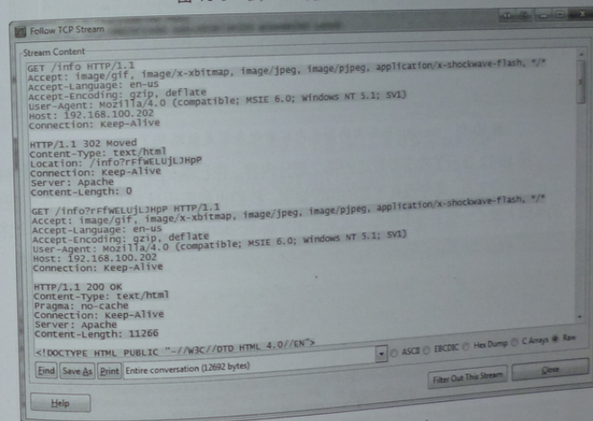
图 10-10 发送到客户端的数据流
