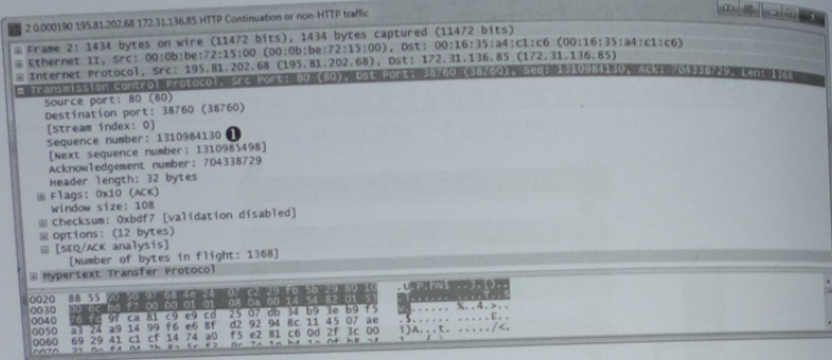
图 9-9 此数据包的序号与预料的不同
