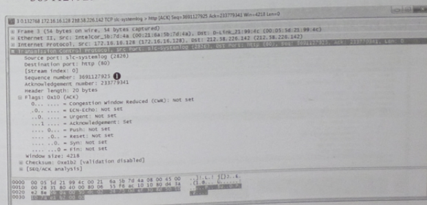
图 6-23 最后的 ACK 包
