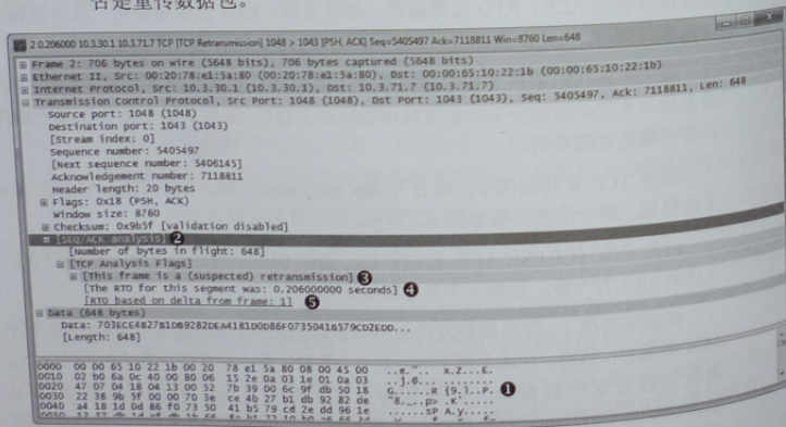
图 9-4 一个重传数据包
