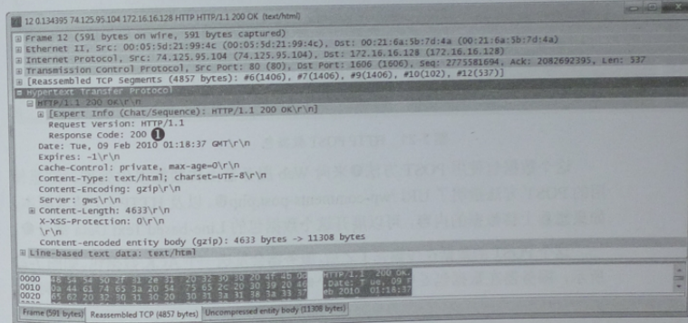
图 7-20 最后有着响应码 200 的 HTTP 数据包
