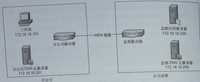
图 8-33 分公司之困问题的相关组件
