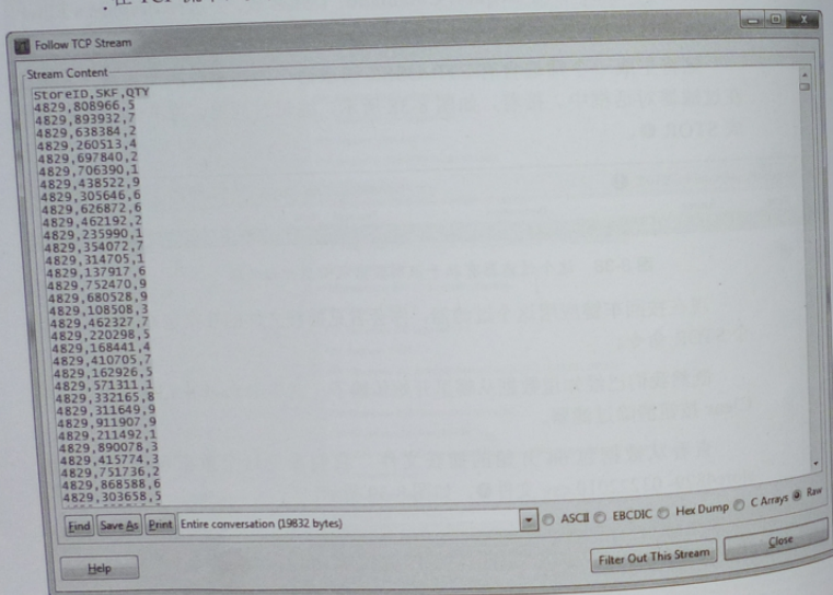
图 8-40 TCP 流显示了传输的数据
