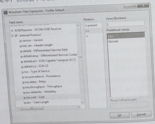
图 4-13 Filter Expression 对话框可以让你很容易地在 Wireshark 中创建过滤器
