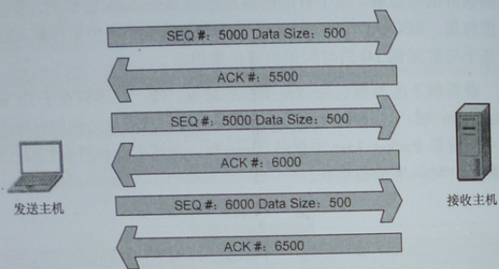
图 9-6 TCP 序号和确认号
