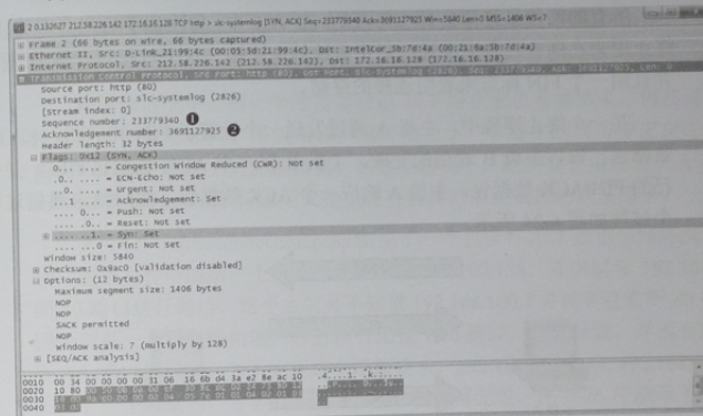
图 6-22 SYN/ACK 响应
