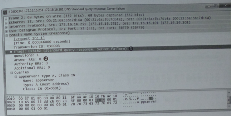
图 8-35 查询响应表明这是上游的问题
