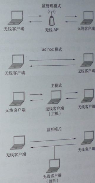
图 11-4 不同的无线网卡模式
