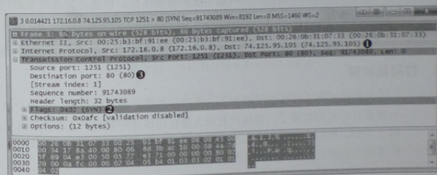
图 8-27 尝试连接 80 端口的 SYN 数据包
