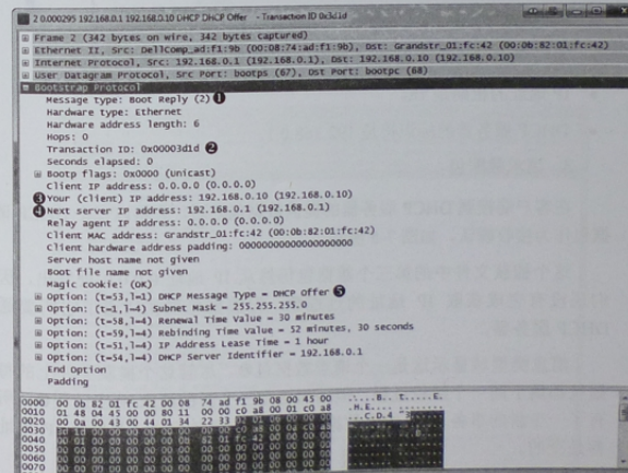
图 7-4 DHCP 提供数据包
