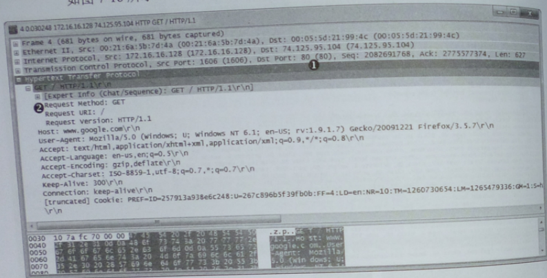
图 7-18 初始 HTTP GET 请求数据包
