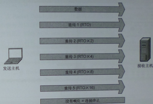
图 9-1 TCP 重传过程的概念视图
