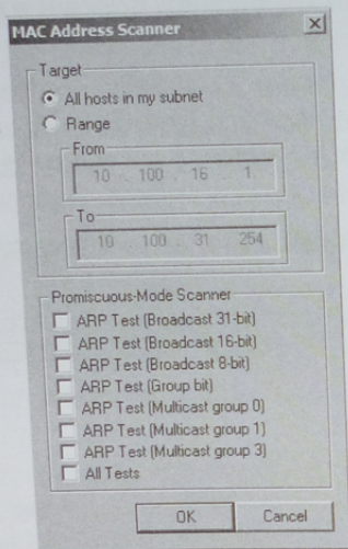
图 2-12 Cain & Abel 网络发现工具
