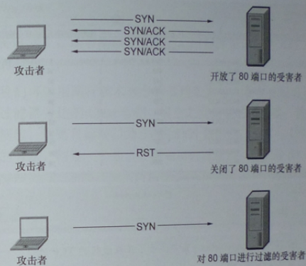
图 10-1 一次 TCP SYN 扫描的结果
