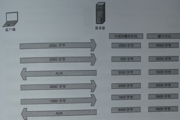
图 9-13 接收窗口使得接收方不被数据淹没
