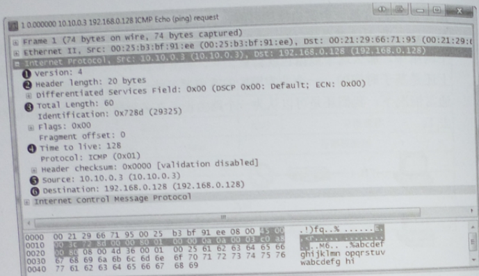
图 6-11 源数据包的 IP 头
