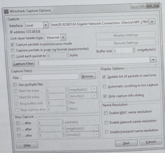
图 4-8 Capture Options 对话框
