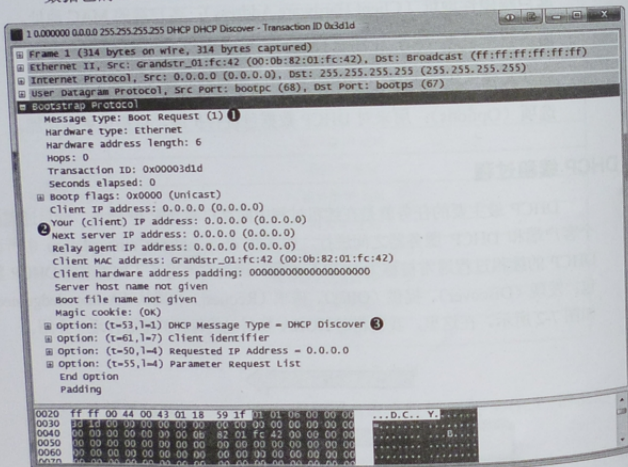
图 7-3 DHCP 发现数据包
