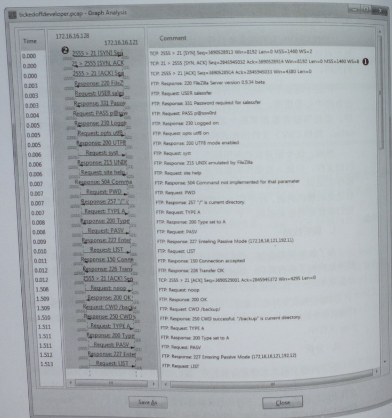
图 8-37 流量图提供了 FTP 通信的快速视图
