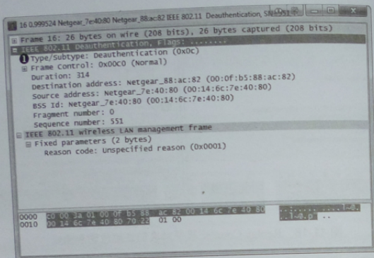
图 11-20 WPA 握手失败后，客户端认证失败
