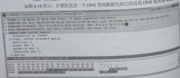
图 8-18 发送到 4.2.2.2 的 DNS 查询
