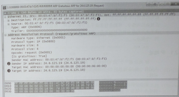
图 6-6 一个无偿 ARP 数据包
