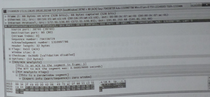
图 9-19 零窗口数据包使数据传输暂停
